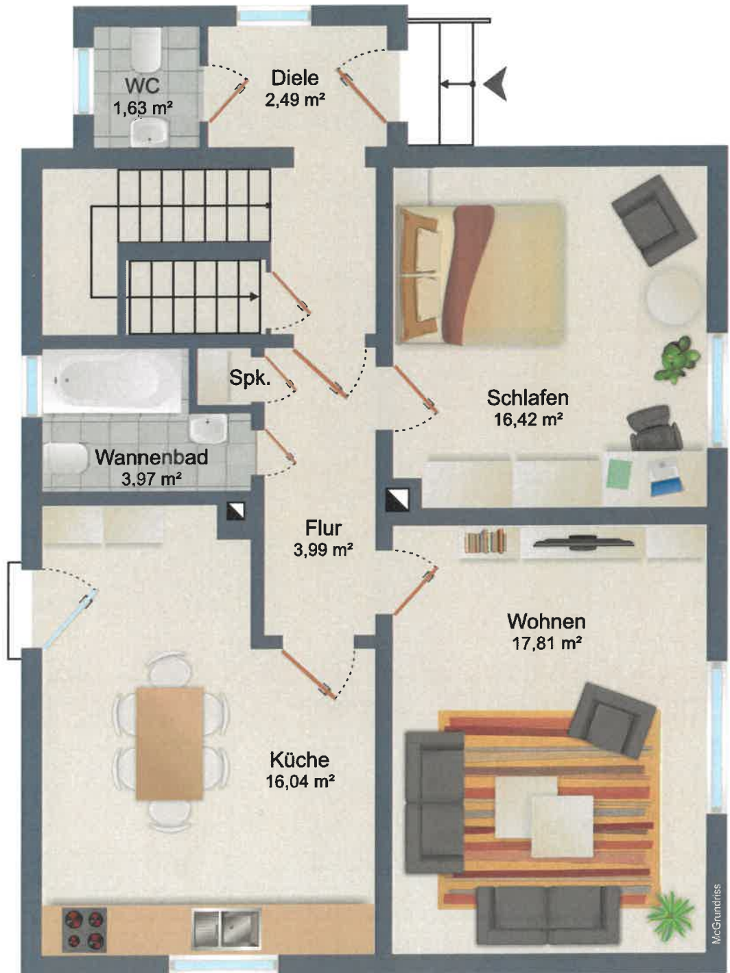
Erdgeschoss
