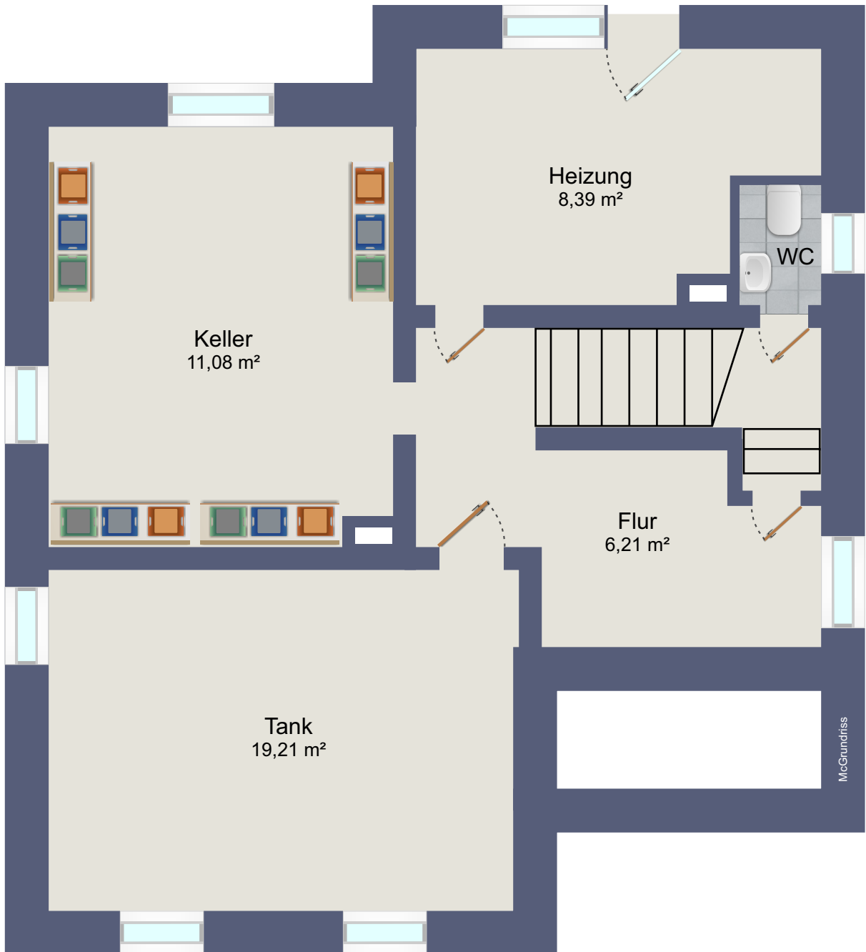
Kellergeschoss
