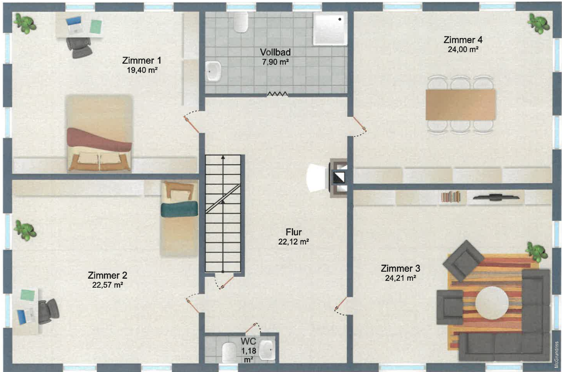
Obergeschoss
